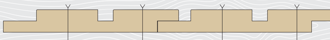
PROFIL NR. 210 – DOBBELTFALSET RETT KLEDNING
