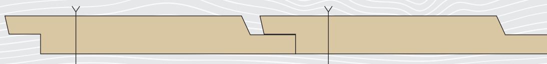
PROFIL NR. 135 – DOBBELTFALSET KLEDNING 60 GRADER NY TYPE
