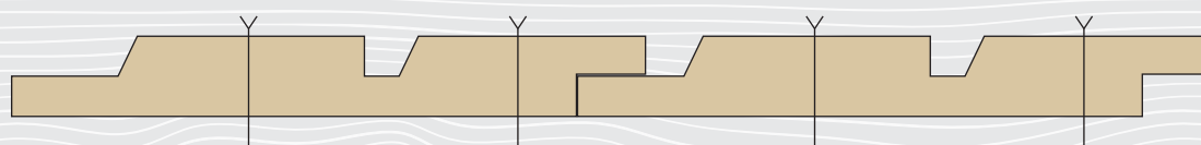
PROFIL NR. 137 – DOBBELTFALSET KLEDNING NY TYPE M/SPOR
